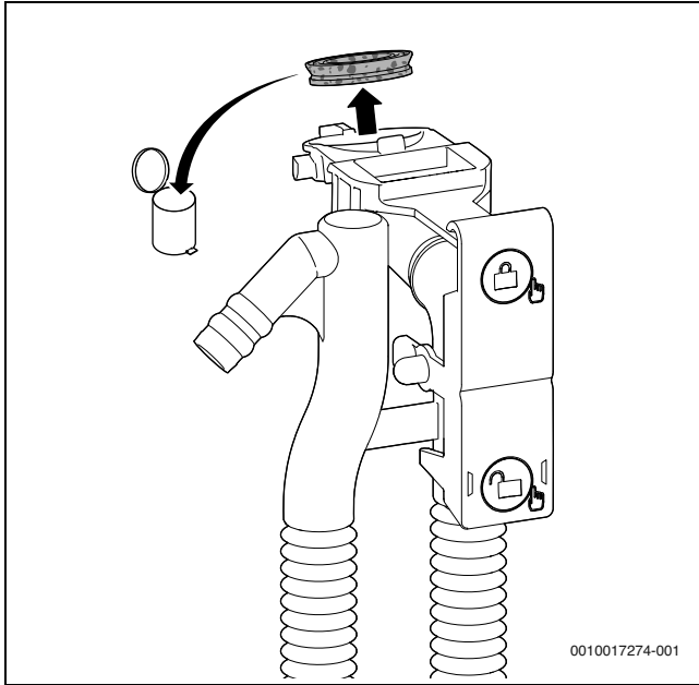
Мал. 59 Заміна ущільнення у верхній частині сифона для відведення конденсату
