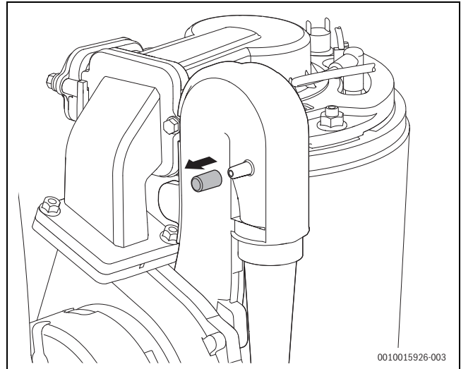
Мал. 47 Штуцер для вимірювання на змішувальній камері
