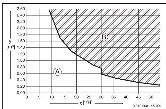
Мал. 26 Вимоги до води для заповнення та підживлення в °fH для приладів потужністю < 50 кВт
