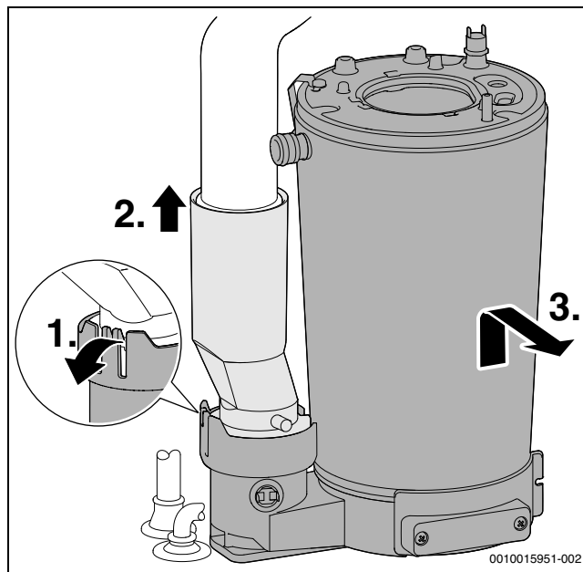
Мал. 72 Демонтаж котлового блоку, який включає камеру згоряння і теплообмінник
