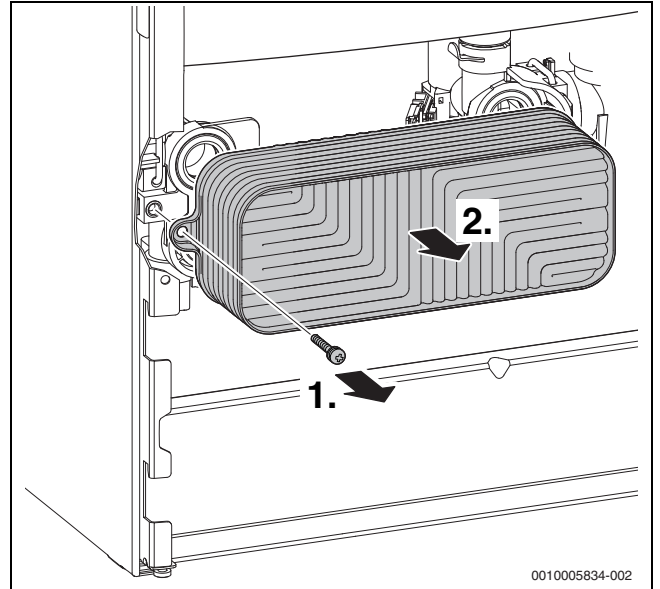
Мал. 65 Демонтаж пластинчастого теплообмінника
