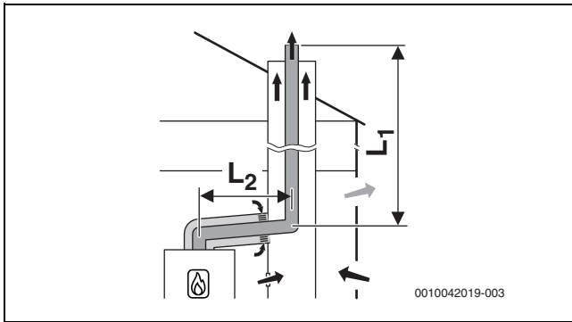
Мал. 16 Система відведення димових газів у шахті жорсткої конструкції згідно з V_{53p} з подачею повітря з приміщення через концентричний з'єднувальний трубопровід у котельному приміщенні; вентиляційний отвір у шахті
