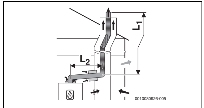
Мал. 18 Система відведення димових газів гнучкої конструкції у шахті згідно з V_{53p} з подачею у прилад повітря з приміщення та трубопроводом з однією стінкою для відведення відпрацьованих газів у котельному приміщенні; вентиляційний отвір у шахті
